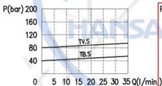
Curve caratteristiche pressione/portata
