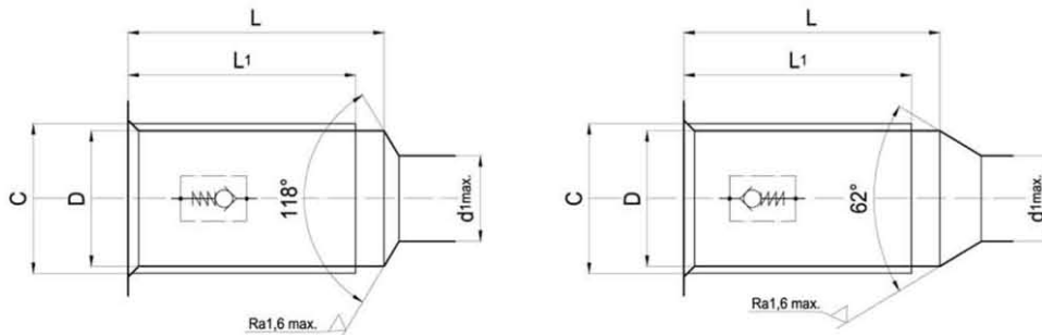
SEDE - CAVITY
